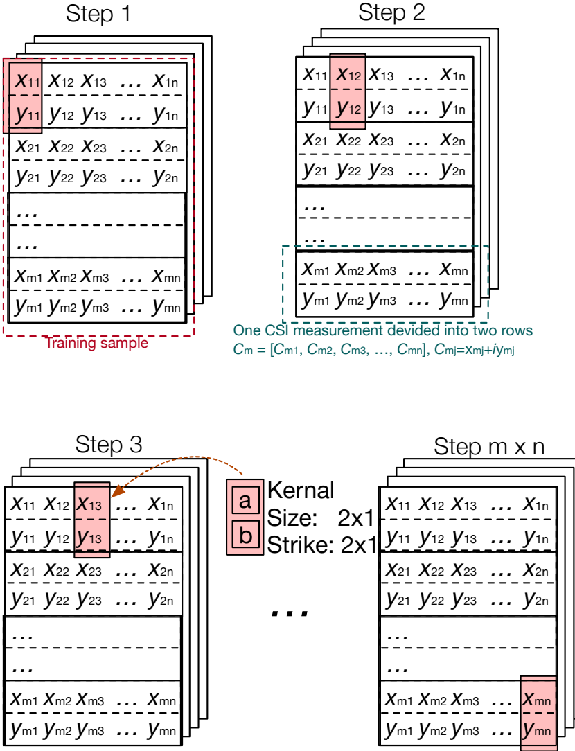
Fig. 7. first layer kernel
